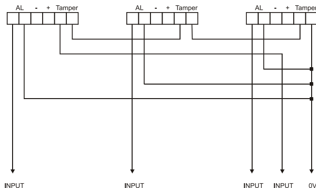
Illustratie 4: detectoren zonder EOL aansluiten
